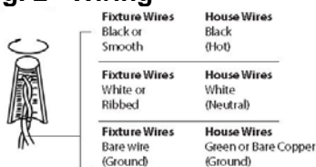
Fig. 2 Wiring
